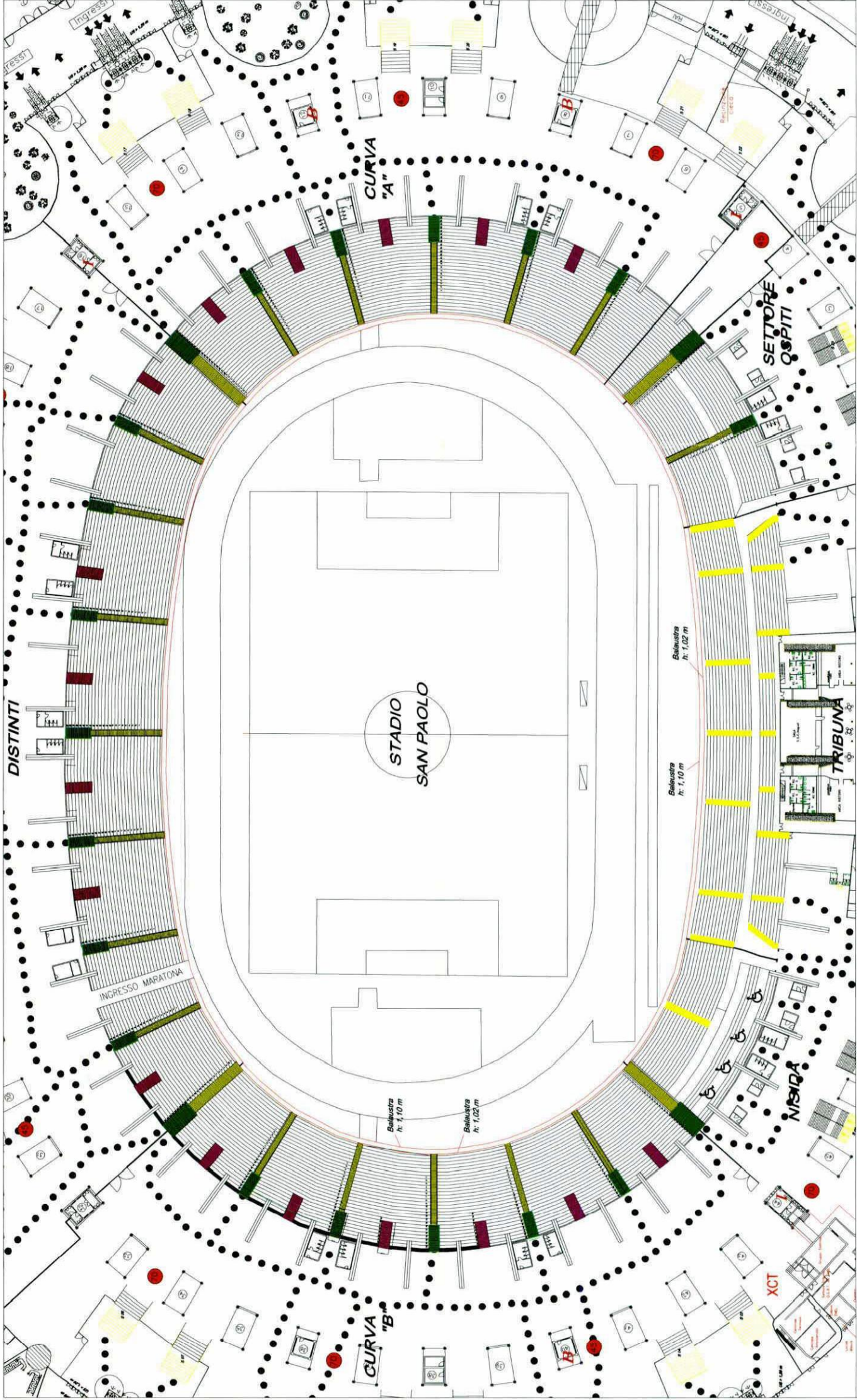
pianta anello inferiore - stato di progetto scala 1:500
