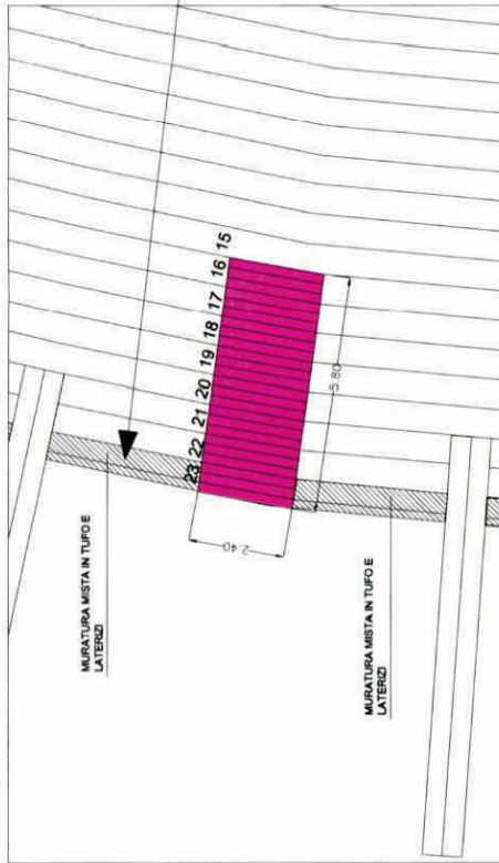
pianta anello inferiore - stato di progetto scala 1:500
